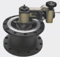
FI355M Flange Facer
